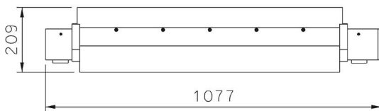
MAGNET DIMENSIONS
